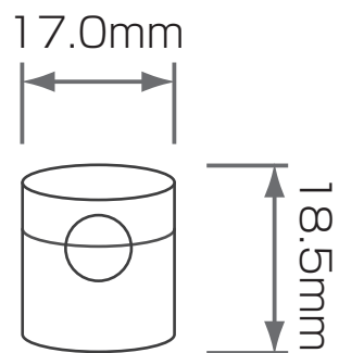
ヒンジキャップ17S
